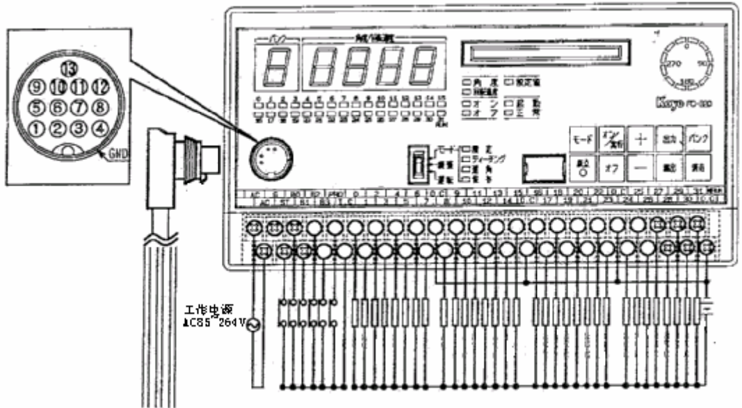
(2) FC-160 的连接配线
