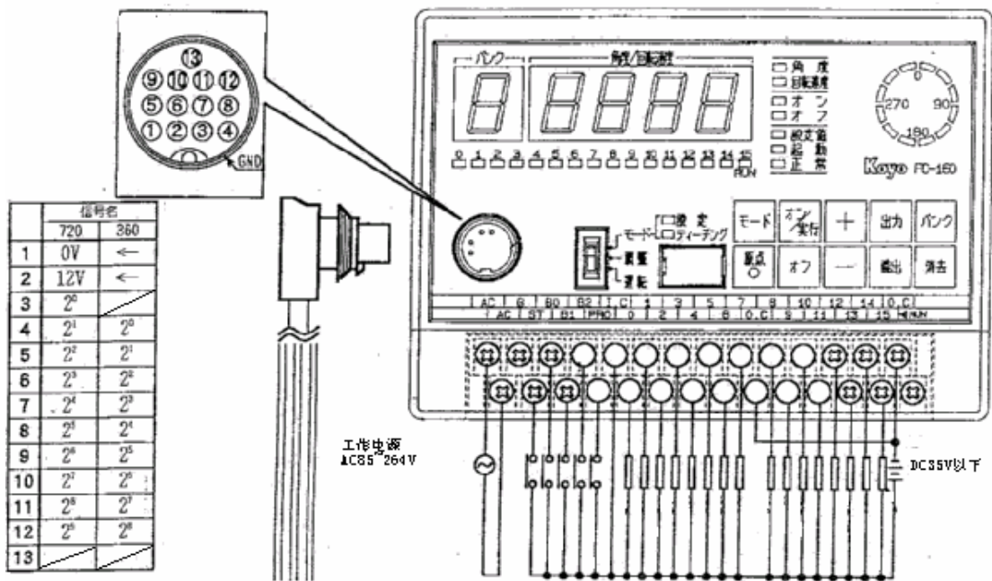
(2) FC-160 的连接配线
