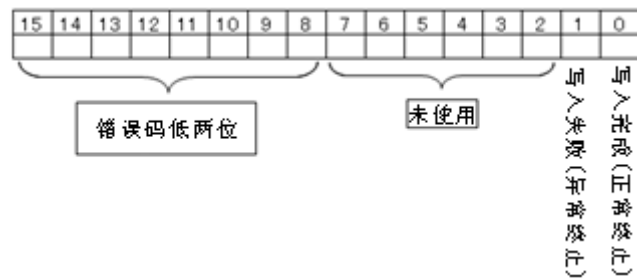
图 10. 保存数 输出存储器
