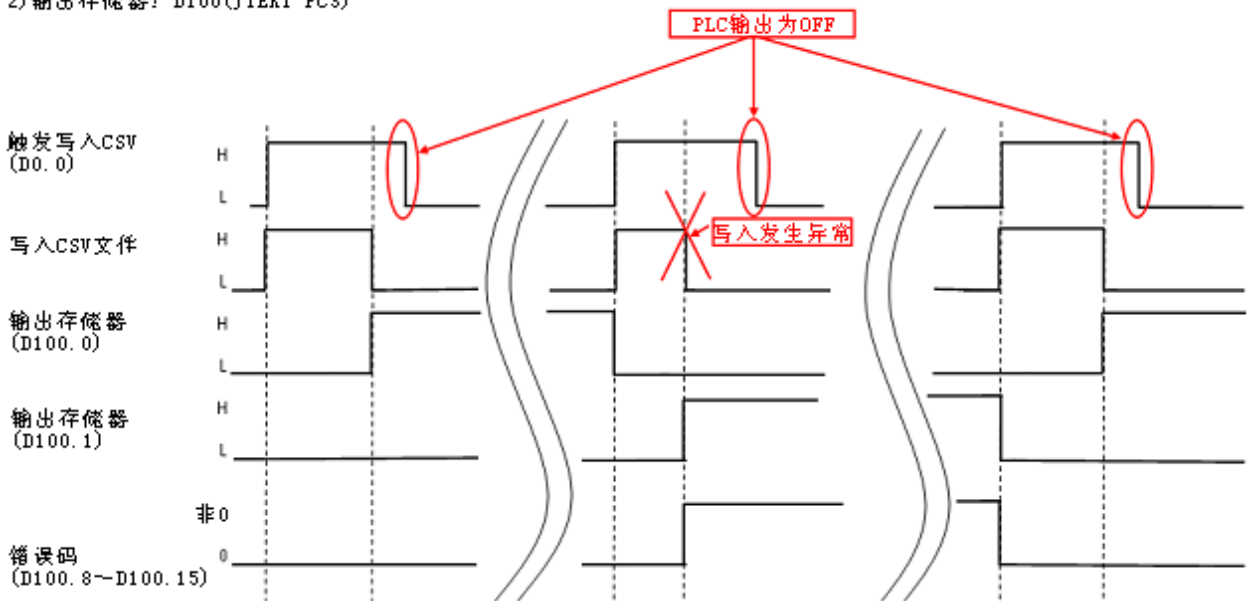
图 11. 输出存储器写入时序
