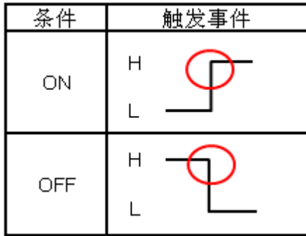
图 8. 用位存储器设置时事件触发条件
