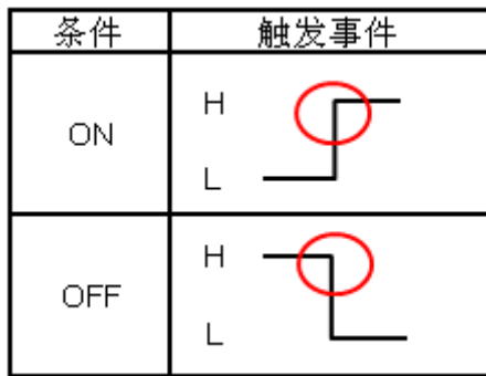
图 6. 用位存储器设置时事件触发条件
