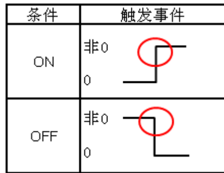
图 7. 用字存储器设置时事件触发条件
