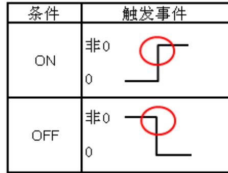
图 9. 用字存储器设置时事件触发条件
